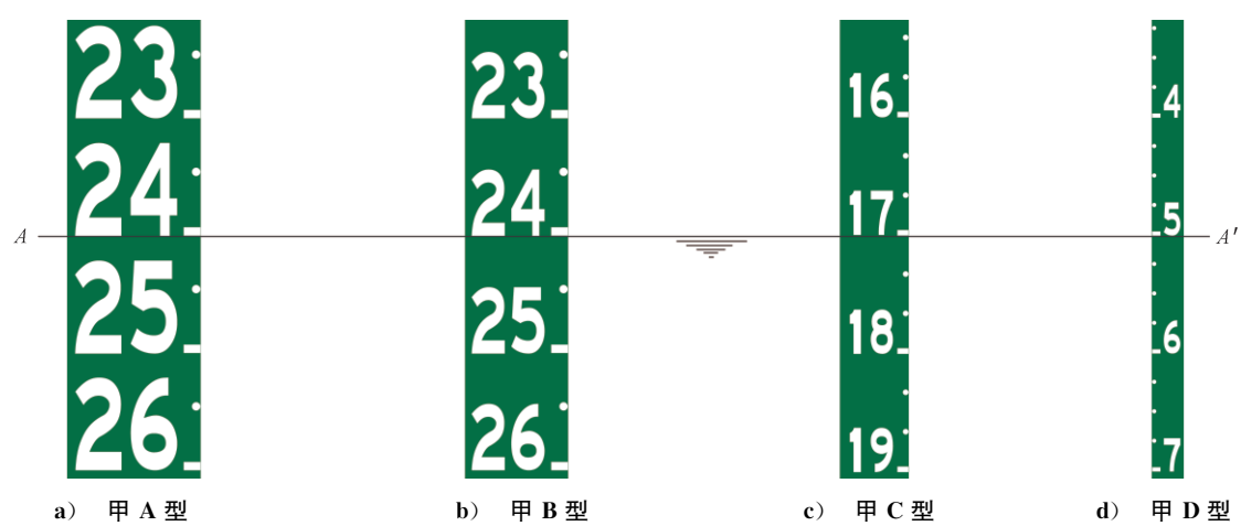
注：当水位在 AA' 时，甲 A 型、甲 B 型标尺显示的实时净空高度为 24 m，甲 C 型标尺为 17 m，甲 D 型标尺为 5 m。
