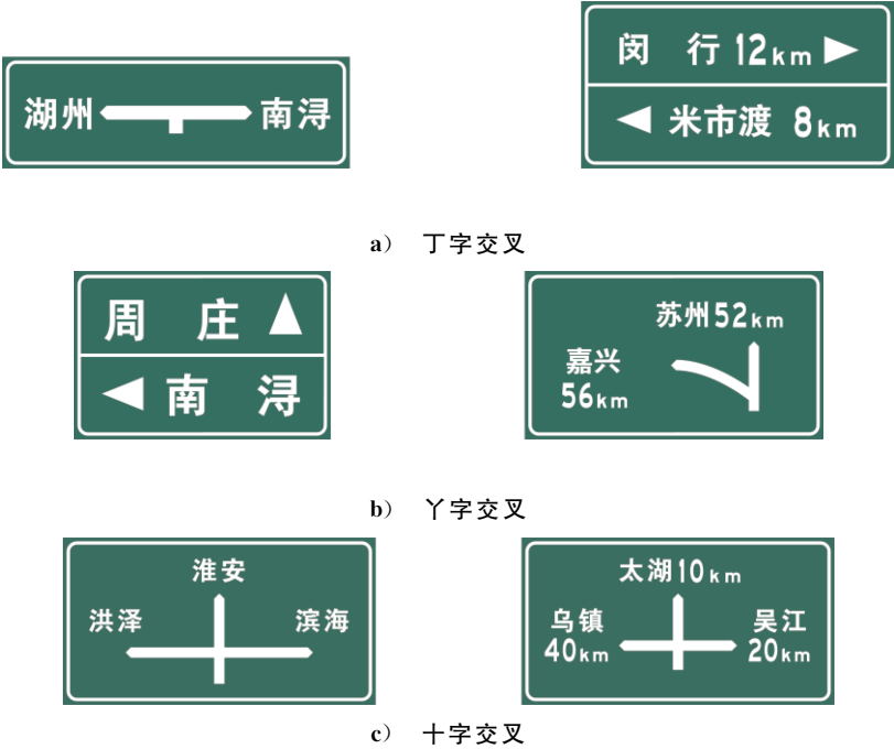
图 70 交叉河口方向距离标志(代码 619)示例
