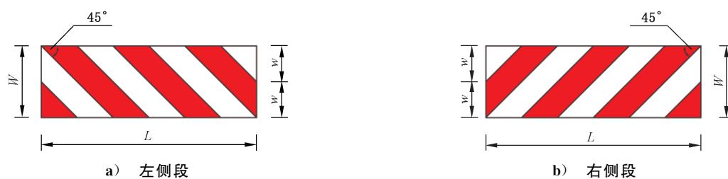
图 81 乙类标志(代码 702)
