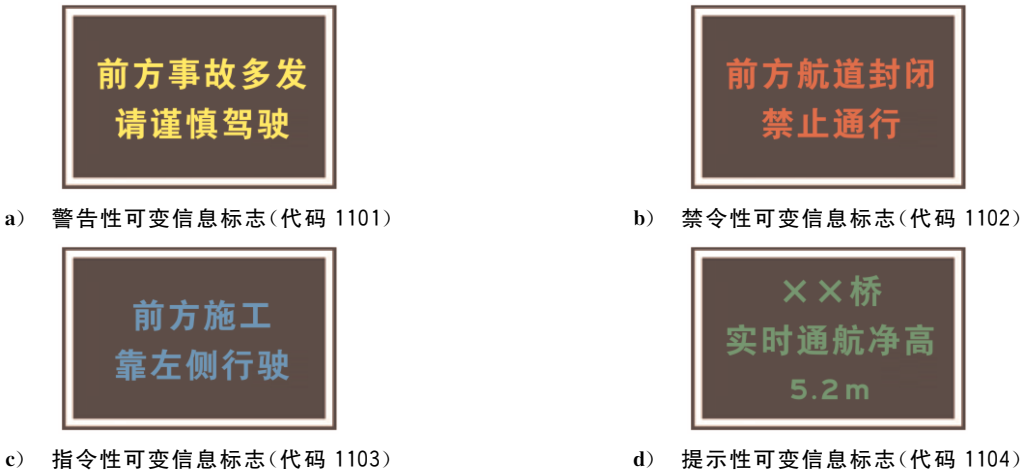
图 88 可变信息标志示例
