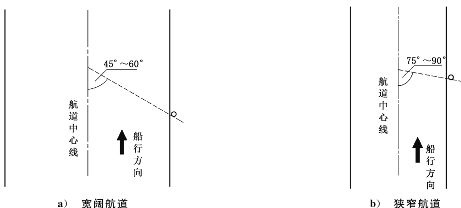
图 89 岸基标志安装角度示意
