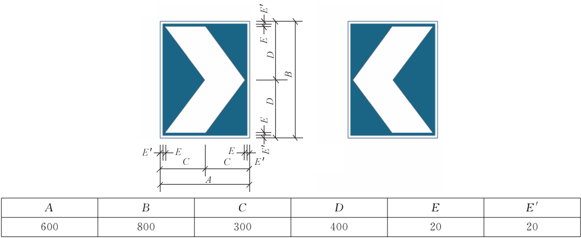
图 48 导向标基本单元(代码 501)
