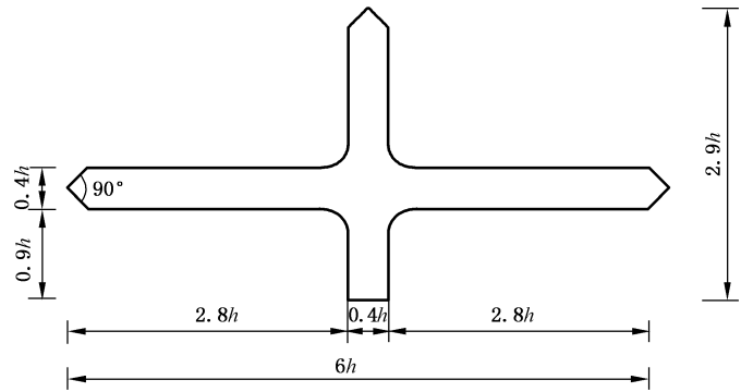
c) 十字交叉(不含距离)图标
